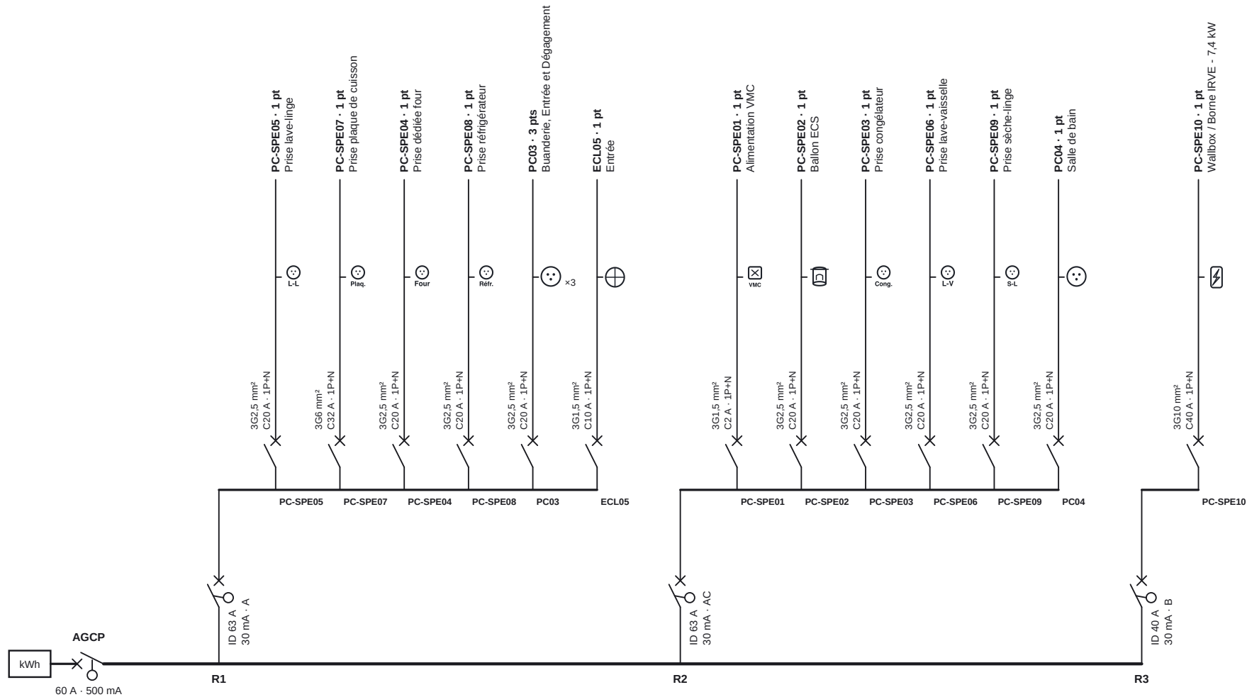
Schéma de distribution - Maison d'exemple - 100 m 2
